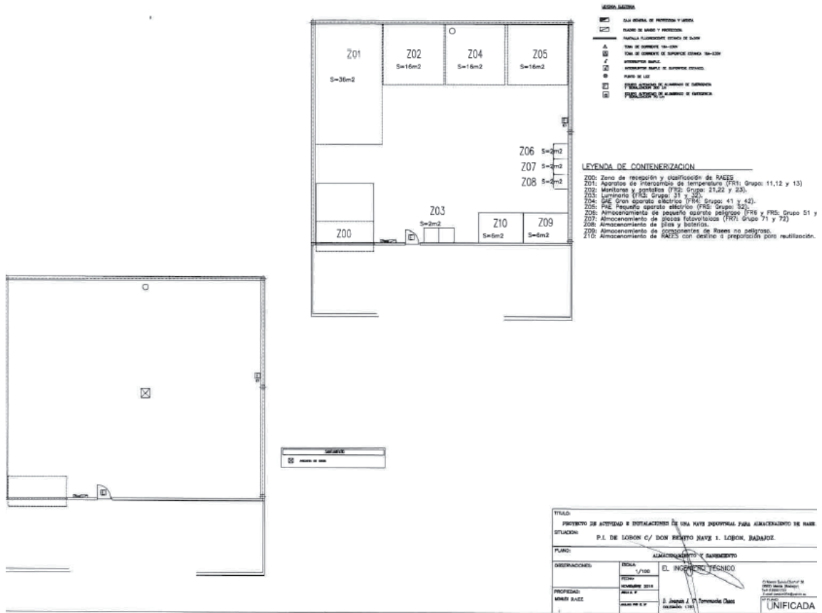
Figura 2. Plano en planta de distribución de las 9 naves.
